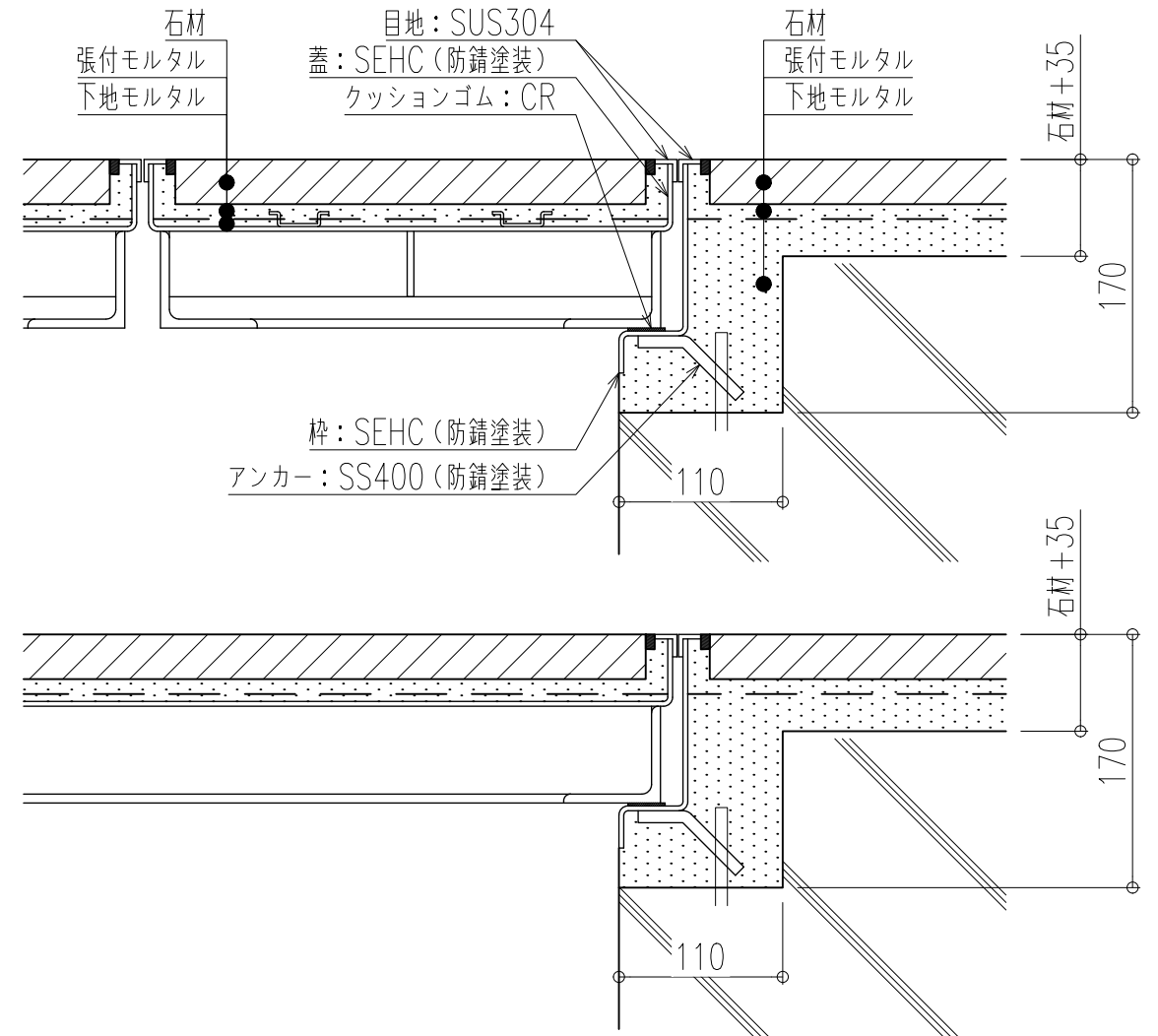
施工参考拡大図
